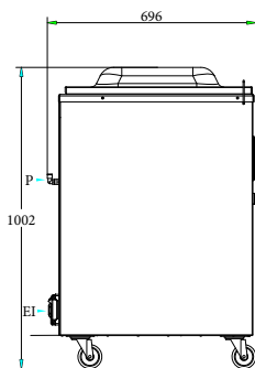
Oldalnézet
