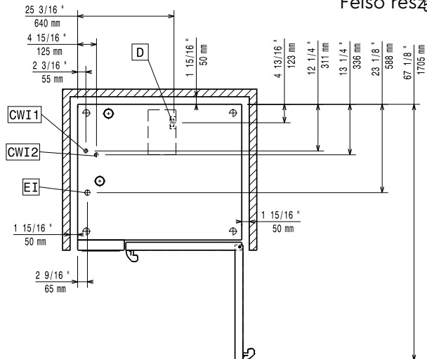
Felső részlet
